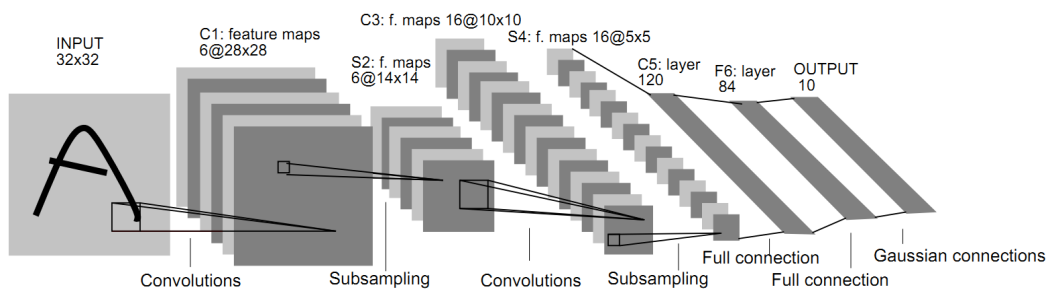
Fig. 2.7.: Schéma du réseau LeNet5, conçu par LeCun et al. [LeC+98] pour la reconnaissance de chiffre manuscrit.
