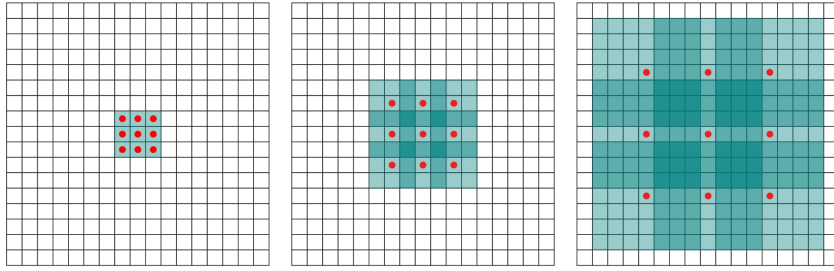
Fig. 4.17.: Champ réceptif des opérateurs de convolutions dilatées utilisant des facteurs de dilatations de 1,2 et 4. Image tirée du papier [YK16].
