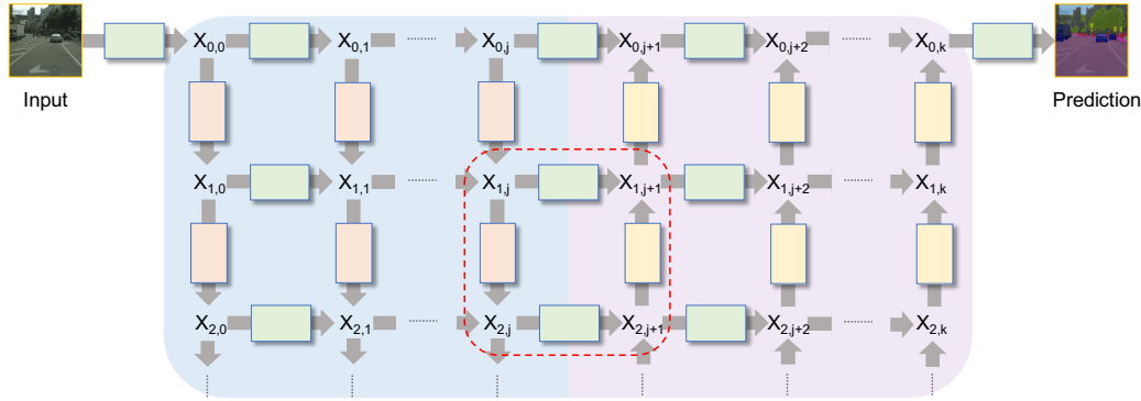
Fig. 6.2.: Schéma de notre réseau GridNet : chaque bloc vert est une unité résiduelle qui ne change ni les résolutions ni le nombre de cartes de caractéristiques d'entrée. Les blocs rouges sont des unités convolutives avec réduction de résolution (sous-échantillonnage) qui doublent le nombre de cartes de caractéristiques. Les blocs jaunes sont des unités déconvolutives qui augmentent la résolution des cartes de caractéristiques et divisent par deux leurs nombres. Un schéma détaillé du carré en pointillé rouge présentant la composition de chacun des blocs est donné dans la figure 6.3
