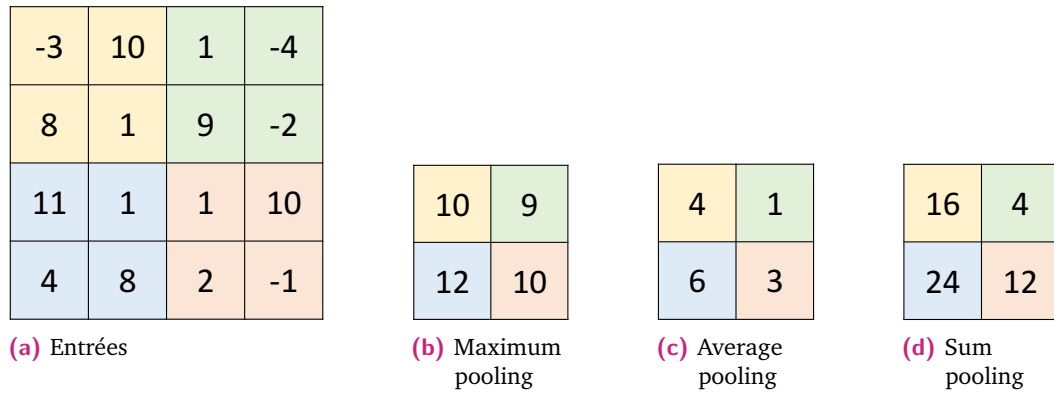
Fig. 2.4.: Exemples de sous-échantillonnages. De gauche à droite : l'entrée, les résultats avec un opérateur de sous-échantillonnage par valeur maximale (maximum pooling), de sous-échantillonnage par valeur moyenne (average pooling) et de sous-échantillonnage par somme (sum pooling).
