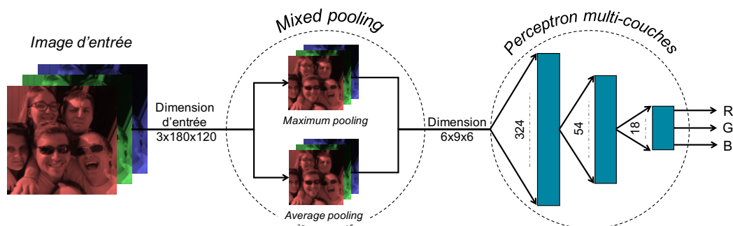
Fig. 3.6.: Notre architecture de réseau de neurones basée sur le sous-échantillonnage mixte avec un support large ( 20 \times 20 ) combiné à un perceptron multi-couches.
