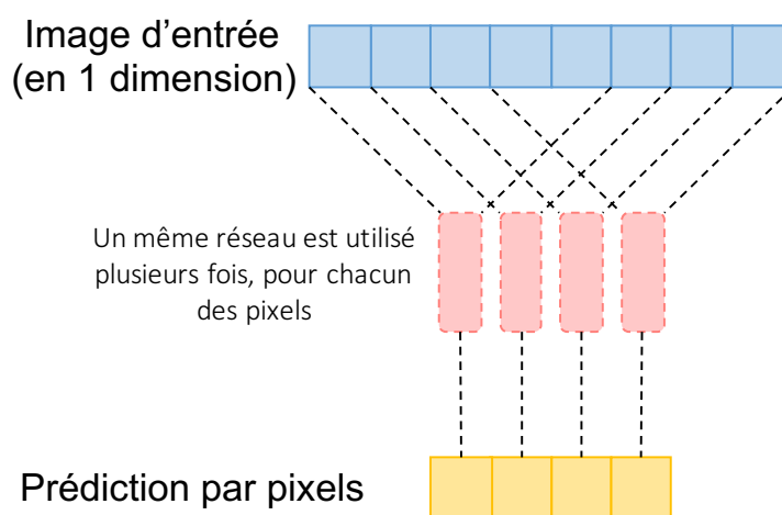
Fig. 4.7.: Méthode naïve pour obtenir une prédiction pour chacun des pixels d'une image d'entrée. Pour des soucis de clarté, l'image (en bleu) n'est représentée en une dimension. Le réseau utilisé, en rouge, est le même pour chaque sous-partie de l'image et prend 5 pixels en entrée. Dans cet exemple les pixels au bord de l'image ne sont pas représentés, mais ils peuvent être annotés en ajoutant des pixels avec une valeur de 0 au bord de l'image.
