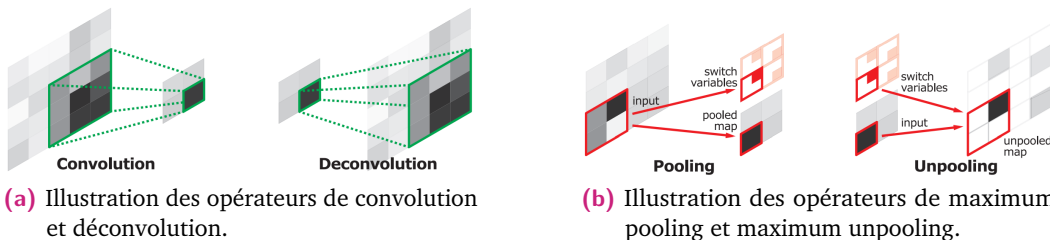
Fig. 4.12.: Opérateurs de convolution et de maximum pooling ainsi que leurs équivalents permettant la reconstruction des cartes de caractéristiques. Image tirée du papier [Noh+15].
