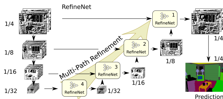
Fig. 4.16.: Schéma du réseau RefineNet [Lin+16b]. Le réseau suit le schéma d'un U-Net mais utilise un opérateur appelé refinenet afin de transformer les cartes de caractéristiques circulant de la partie convolutive à la partie déconvolutive. Image tirée du papier [Lin+16b].
