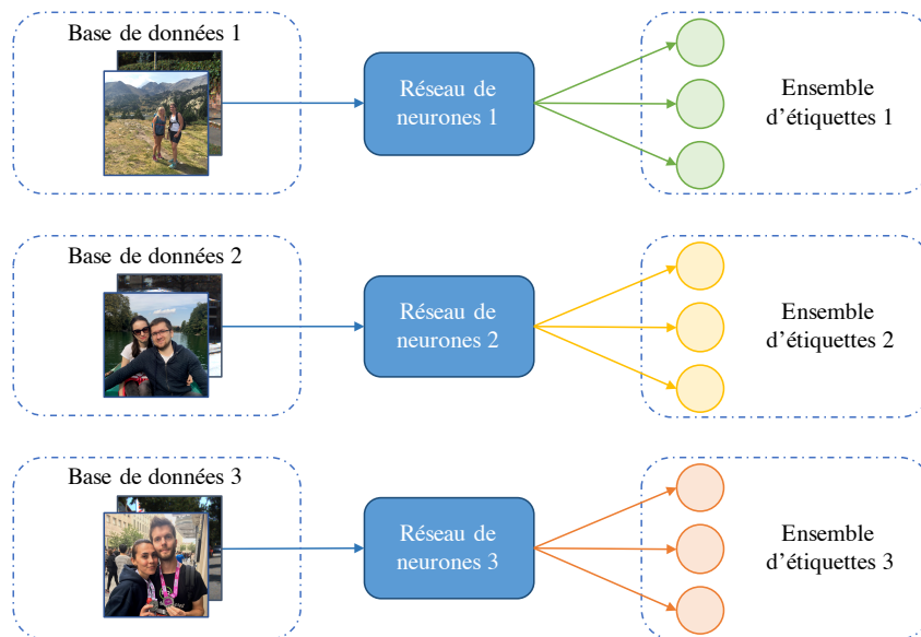
Fig. 5.1.: Stratégie d'apprentissage classique appelée " Baseline ". Elle consiste à entraîner un réseau de neurones par base de données (et ensemble d'étiquettes) différents.
