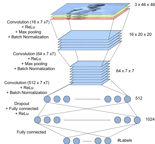
(a) Schéma du réseau utilisé pour nos expérimentations
