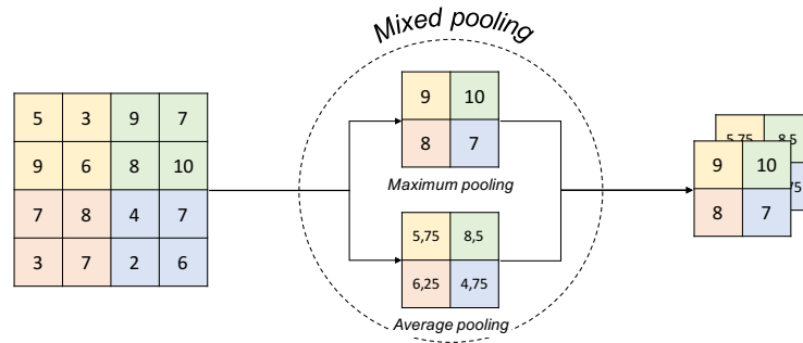
Fig. 3.5.: Illustration de notre sous-échantillonnage mixte. La fenêtre d'observation est de 2 \times 2 .
