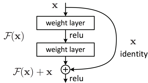
Fig. 2.13.: Illustration d'une couche résiduelle [He+16a]. L'entrée est additionnée aux résultats du mapping. Figure extraite du papier d'origine [He+16a]
