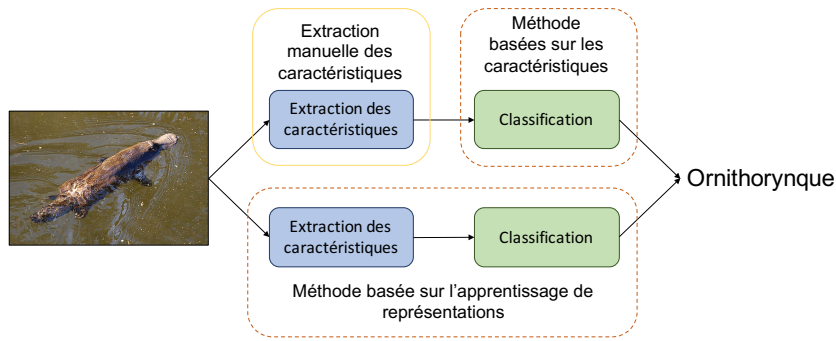
Fig. 1.1.: Illustration de la différence entre les méthodes basées sur les caractéristiques (chemin du haut) et les méthodes basées sur l'apprentissage de représentations (en bas). Les rectangles en pointillés montrent les parties entraînées par les algorithmes.
