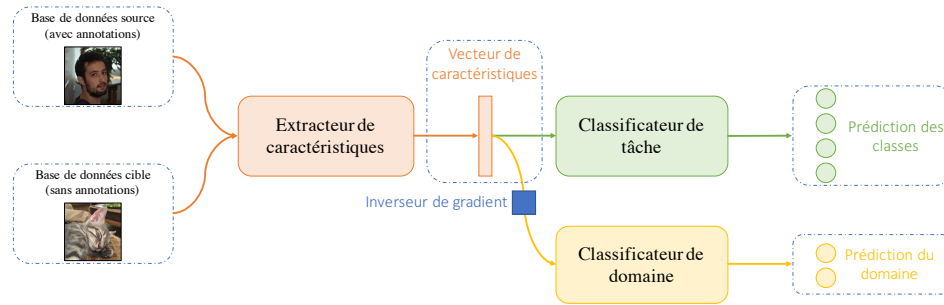
Fig. 5.4.: Illustration de l'inverseur de gradient de Ganin et Lempitsky [GL15]. L'extracteur de caractéristiques (en orange) extrait des caractéristiques utilisées par les deux classificateurs. Le classificateur de tâche (en vert) est entraîné à prédire les classes des images venant de la base de données source. Le classificateur de domaine (en jaune) est entraîné à prédire la provenance des images (base de données source ou base de données cible). L'inverseur de gradient (en bleu) inverse le gradient qui remonte du classificateur de domaine ayant pour effet d'entraîner l'extracteur de caractéristiques à extraire des données invariantes aux bases de données source et cible.
