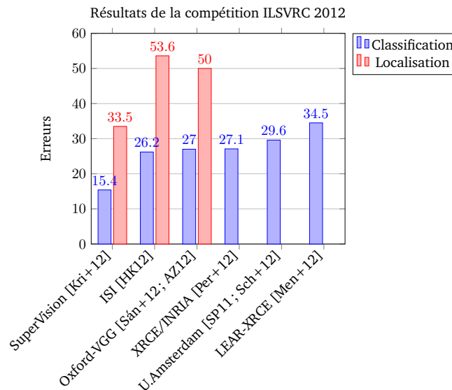
Fig. 2.8.: Résultats de la compétition ILSVRC 2012 [Rus+15] obtenus par les cinq meilleures méthodes.
