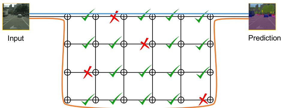
Fig. 6.5.: Le chemin bleu, qui utilise uniquement les connexions hautes résolutions, est plus court que le chemin orange qui utilise un chemin à basse résolution. Afin de forcer le réseau à utiliser tous les chemins de manière équivalente, nous coupons aléatoirement des chemins lors de l'entraînement, tel qu'illustré par les croix rouges.
