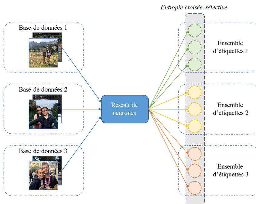
Fig. 5.2.: "Apprentissage Joint" (AJ) d'un unique réseau utilisant notre fonction d'entropie croisée sélective.
