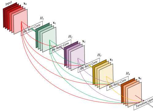
Fig. 2.15.: Illustration d'un bloc dense de 5 couches avec un facteur de croissance de 4. Schéma tiré du papier [Hua+16b]
