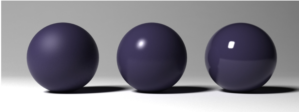
Fig. 3.2.: La sphère à gauche possède une réflexion diffuse tandis que la sphère à droite a une réflexion spéculaire. La sphère du milieu est une combinaison entre réflexion diffuse et spéculaire.
