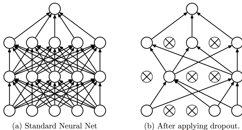
Fig. 2.6.: Illustration de l'opérateur de Dropout (tirée du papier [Sri+14]). À droite le réseau entièrement connecté. À gauche, des neurones ont été aléatoirement désactivés.
