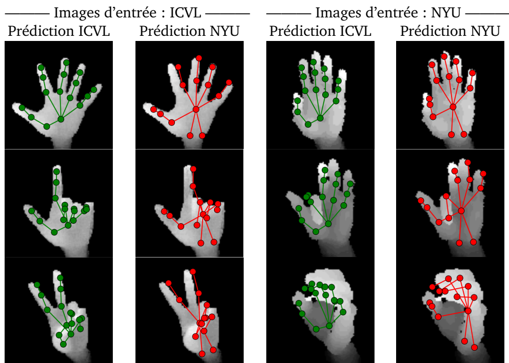
Fig. 5.10.: Résultats de la stratégie apprentissage joint avec partage de contexte appliquée à la tâche d'estimation de la pose de la main. Les images des deux colonnes de gauche sont tirées de la base de données ICVL [Tan+13] et les images des deux colonnes de droites proviennent de la base de données NYU [Tom+14].
