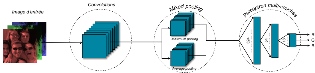
Fig. 3.7.: Architecture de réseau de neurones convolutif. L'image est passée dans une couche de convolutions, suivie de notre sous-échantillonnage mixte et enfin fourni à un perceptron multi-couches.
