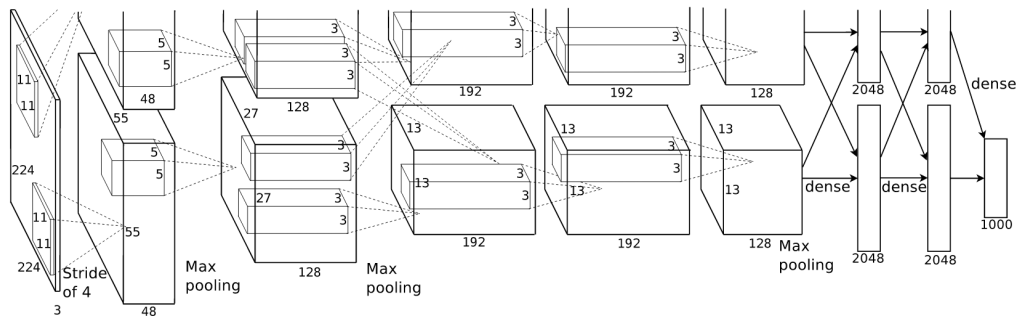
Fig. 2.9.: Schéma du réseau AlexNet. Figure extraite du papier d'origine [Kri+12].
