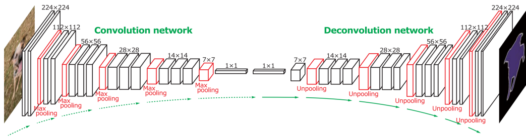
Fig. 4.11.: Réseau Conv-Deconv utilisé par Noh et al. Le réseau est composé de deux parties : une partie convolutive (à gauche) et une partie déconvolutive symétrique (à droite). Dans leurs expériences, ils utilisent un réseau de type VGG16 pour la partie convolutive. Image tirée du papier [Noh+15]
