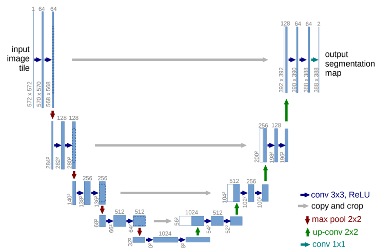
Fig. 4.15.: U-Network. Les cartes de caractéristiques extraites avant les opérateurs de sous-échantillonnage de la partie convolutive sont concaténées aux cartes de caractéristiques extraites après les opérateurs de sur-échantillonnage de la partie déconvolutive. Image tirée du papier [Ron+15].
