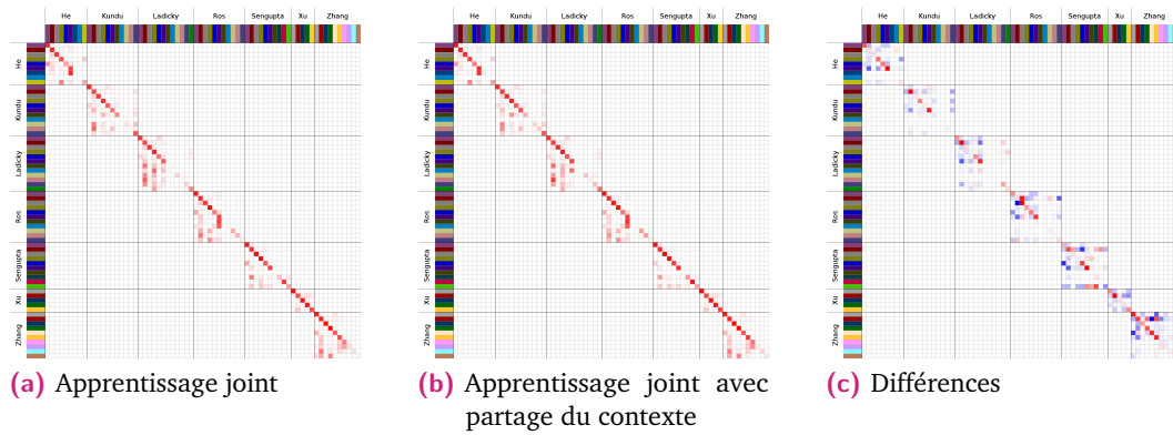
Fig. 5.9.: Matrices de confusion obtenues avec nos stratégies d'apprentissage joint 5.9a et d'apprentissage joint avec partage du contexte 5.9b ainsi que la différence entre les deux 5.9c. Les matrices sont normalisées par lignes et l'intensité des couleurs montre les valeurs les plus élevées. Les valeurs en bleue sont négatives et en rouge positives. Les 68 lignes/colonnes correspondent aux 68 étiquettes détaillées dans le tableau 5.6.
