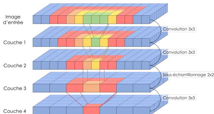
Fig. 4.6.: Illustration du champ réceptif d'un réseau de convolution. Au fil des opérations de convolutions, la zone visible de l'image d'entrée est de plus en plus large.
