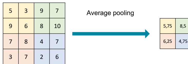
Fig. 3.3.: Exemple d'average pooling avec une fenêtre d'observation de 2 \times 2 .
