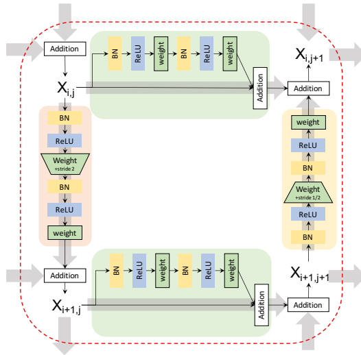
Fig. 6.3: Schéma détaillé des blocs composant notre GridNet. Les unités vertes sont résiduelles et gardent les dimensions des cartes de caractéristiques constantes entre l'entrée et la sortie. Les unités rouges sont convolutives. La partie "weight" en forme de losange est une couche convolutive avec un pas de deux, réduisant ainsi la résolution des cartes de caractéristiques et doublant leurs nombres. Les unités jaunes sont déconvolutives et doublent la résolution des cartes de caractéristiques avec une convolution stridée d'un pas d'un demi. BN = normalisation par batch.
