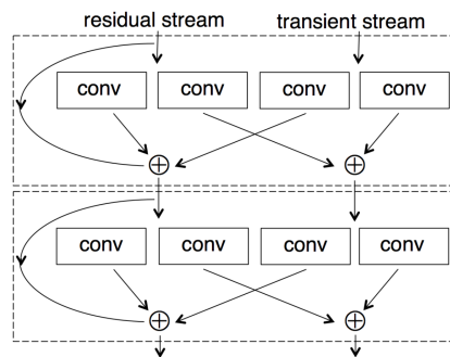
Fig. 2.14.: Illustration de deux couches RiR (ResNet in ResNet) consécutives. Schéma tiré du papier [Tar+16]
