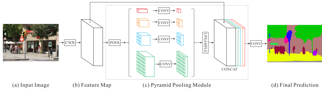
Fig. 4.18.: Illustration du réseau PSPNet (Pyramid Scene Parsing Network) de Zhao et al. [Zha+16]. La sortie d'un ResNet spécialisé à la segmentation sémantique est sous-échantillonnée à plusieurs résolutions avant d'être traitées par plusieurs convolutions. Un opérateur reconstruit ensuite les cartes de caractéristiques leur permettant d'être concaténées et utilisées par une dernière convolution fournissant la prédiction. Cette image est tirée du papier [Zha+16].
