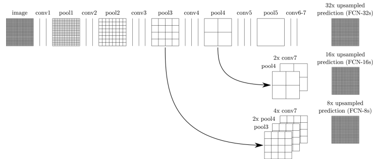
Fig. 4.10.: Des convolutions sont utilisées pour reconstruire les cartes de caractéristiques et augmenter la taille de la prédiction finale. Afin de permettre une meilleure reconstruction, les cartes de caractéristiques extraites dans les parties convolutives sont aussi utilisées. Image tirée du papier [Lon+ 15].
