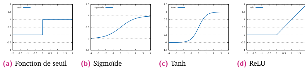
Fig. 2.2.: Les fonctions d'activations les plus connues. De gauche à droite : la fonction de seuil (historique mais inutilisable dans les réseaux d'aujourd'hui), Sigmoide, Tanh et ReLU (Rectified Linear Unit).
