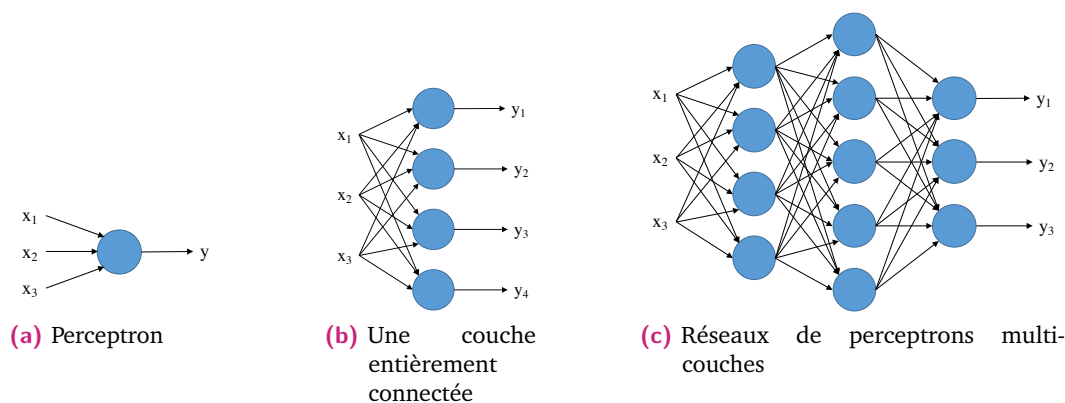
Fig. 2.1.: Différentes étapes de construction d'un réseau de perceptrons multi-couches. À gauche, l'unité de base des réseaux de neurones : un perceptron. Au milieu, plusieurs perceptrons sont utilisés en parallèle pour former une couche entièrement connectée. À droite, plusieurs couches sont utilisées les unes à la suite des autres pour former un réseau de perceptrons multi-couches
