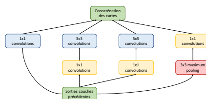
Fig. 2.12.: Module d'inception du réseau GoogleNet [Sze+15a]. Le module est composé de quatre chemins en parallèle, utilisant des convolutions avec des masques de tailles différentes.
