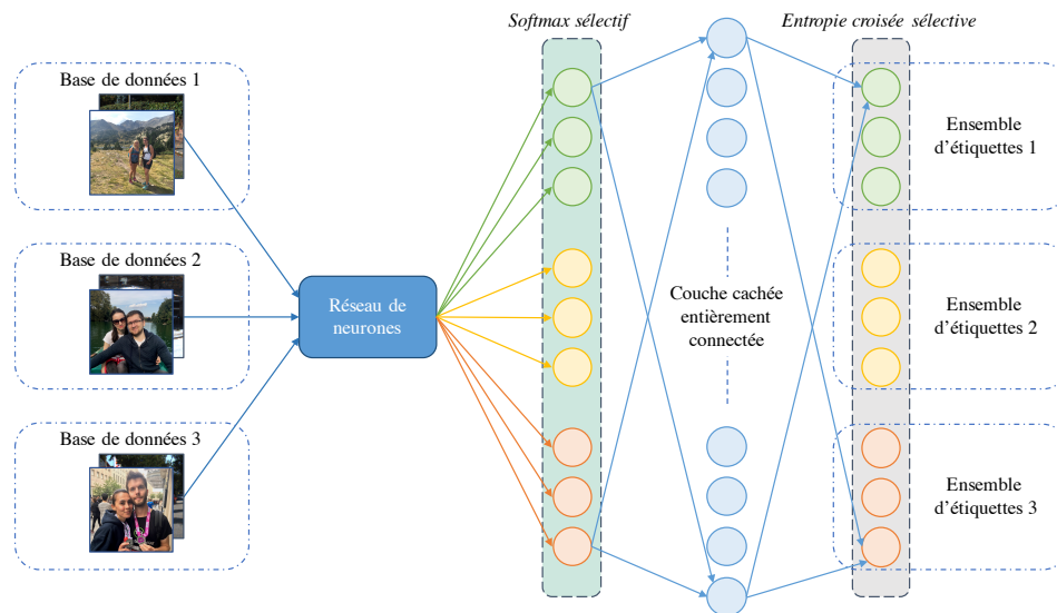
Fig. 5.3.: "Apprentissage joint avec partage de contexte" (AJPC). On ajoute une couche entièrement connectée (MLP) après la sortie d'un premier réseau, pré-entraîné avec la stratégie d'apprentissage joint (figure 5.2). Une deuxième phase d'apprentissage est ensuite réalisée afin de prendre en compte les corrélations entre les classes sémantiques des différents ensembles d'étiquettes.
