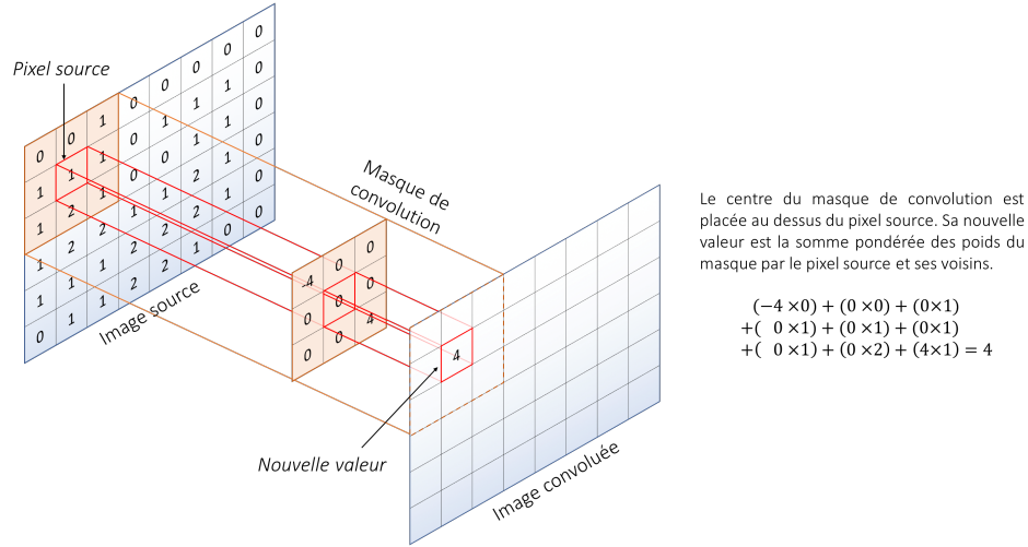
Fig. 2.3.: Illustration d'un opérateur de convolution. L'image source est convoluée avec un masque de convolution (ici de taille 3 \times 3 ). Il est important de noter que, pour l'illustration, le masque de convolution a subi une rotation verticale et horizontale.
