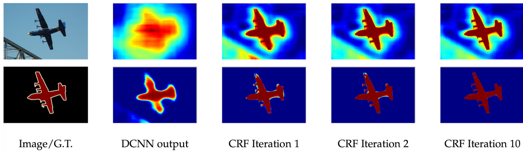
Fig. 4.19.: Exemple d'amélioration obtenue grâce à l'utilisation de CRF. La première ligne montre les valeurs obtenues avant la couche de softmax et la deuxième ligne les valeurs obtenues après le softmax. Image tirée du papier [Che+14a].
