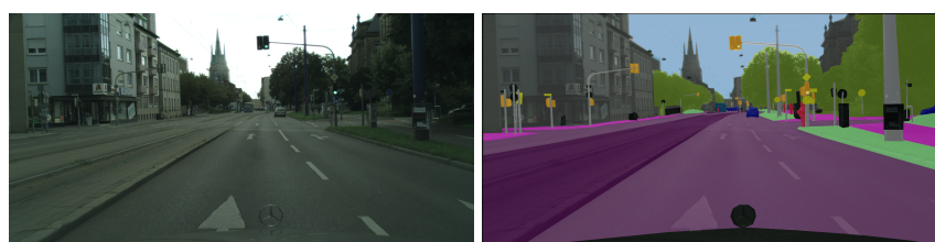
(a) Exemple d'entraînement avec annotations denses
