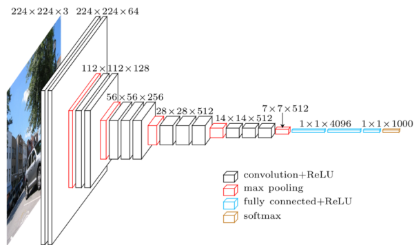
Fig. 2.10.: Schémas du réseau VGG16. Image tirée de la présentation de Matthieu Cord.
