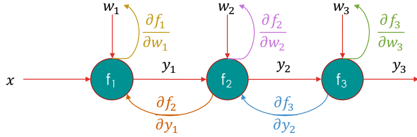
Fig. 2.5.: Exemple du calcul de gradient sur un réseau composé de trois opérateurs f_1 , f_2 , f_3 dépendant des paramètres w_1 , w_2 et w_3 .
