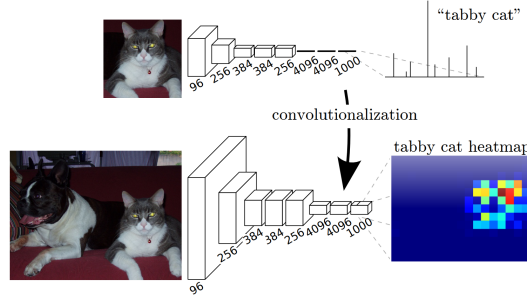
Fig. 4.9.: Les parties entièrement connectées d'un réseau peuvent être transformées en couche convolutives permettant d'utiliser des sorties à différentes tailles. Image tirée du papier [Lon+15].
