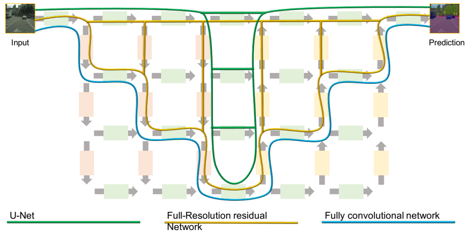
Fig. 6.4.: GridNet généralise plusieurs réseaux classiques, spécialisés pour la segmentation sémantique, tels que les réseaux Conv-Deconv (chemin bleu) (voir 4.3.3), les U-Networks (Chemin Vert) (voir 4.3.4) et le Full Resolution Residual Networks (FRRN) (chemin jaune).
