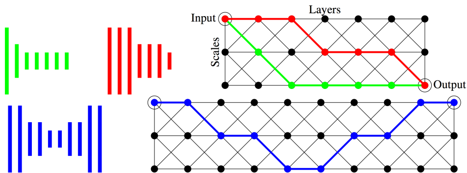
Fig. 6.1.: Schémas des Neural Fabrics de Saxena et al. [SV16]. Leurs structures sont très similaires à notre GridNet et permettent de généraliser des réseaux traditionnels, tel que des réseaux convolutifs à 7 couches (en rouge et vert) et des réseaux conv-déconv à 10 couches (en bleu).
