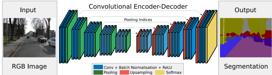
Fig. 4.13.: Schémas du réseau SegNet [Bad+15] développé par Badrinarayanan et al. L'architecture de ce réseau est très proche de celle de Noh et al. illustrée dans la figure 4.11 mais ne possède pas de partie entièrement connectée. Image tirée du papier [Bad+15].
