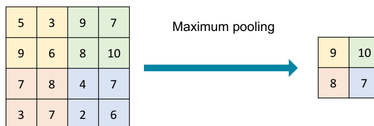
Fig. 3.4.: Exemple de maximum pooling. La fenêtre d'observation est de 2 \times 2 .
