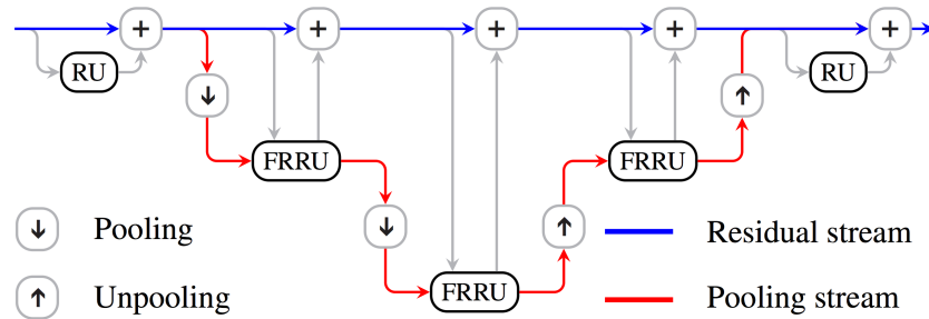
Fig. 4.14.: Schémas du réseau Full Resolution Residual Network (FRRN) de Pohlen et al. [Poh+16]. Le réseau est composé de deux réseaux interconnectés, un réseau conv-deconv (en rouge) et un réseau résiduel (en bleu). Des opérateurs de redimensionnement sont utilisés pour connecter les deux (en gris). La figure est tirée du papier d'origine [Poh+16].
