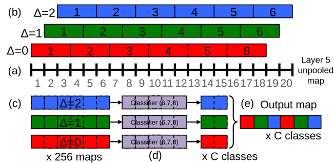
Fig. 4.8.: Illustration en 1 dimension. L'image représentée par le tableau (a) est décalée trois fois (b) pour être passée dans trois opérateurs de sous-échantillonnages (b). Les résultats obtenus (c) sont donnés au classificateur (d). Les résultats finaux sont ensuite ordonnés (e) permettant d'obtenir une sortie plus dense. L'image est tirée du papier d'origine [Ser+13]
