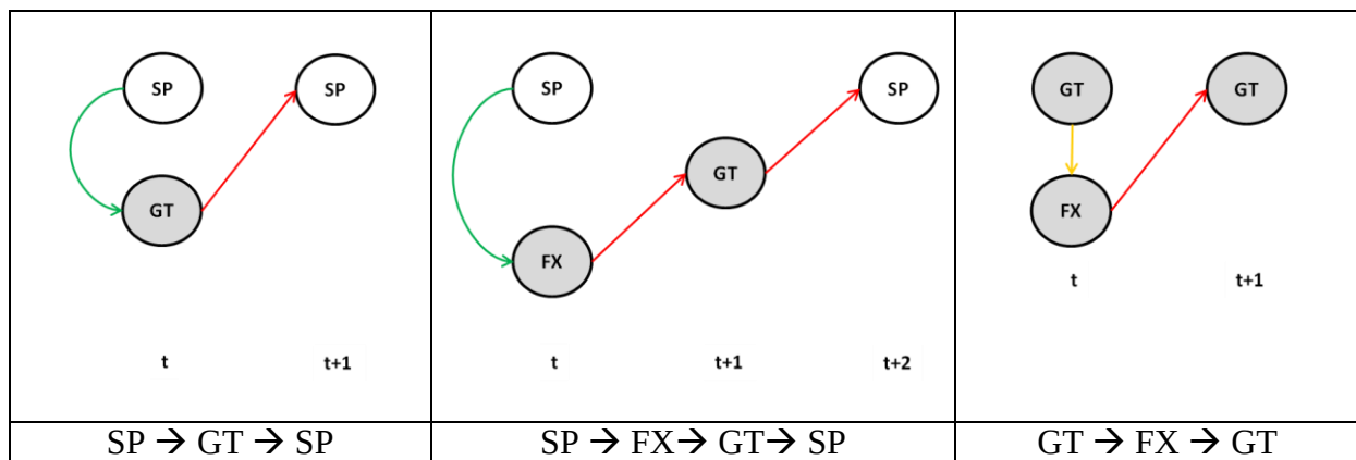
Figure 70 : Propriété 3 (inter-slices)
