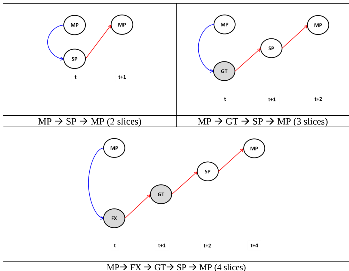
Figure 69: Propriété 2 (inter-slices)
